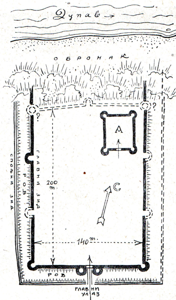
Сл. 6 — Скица основе римског кастрома код Рама — Plan du castrum près de Ram
